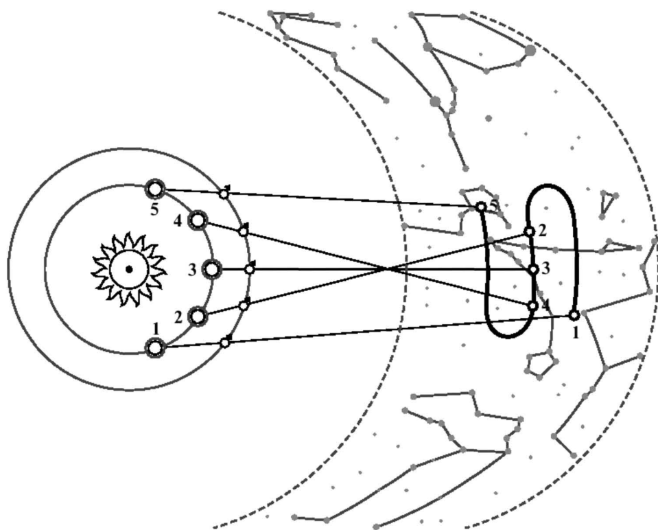
Рис. 5. Земля, двигаясь по ближней к Солнцу орбите, «обгоняет» планету (например, Марс), движущуюся по дальней орбите. Для наблюдателя с Земли будет казаться, что на некоторое время Марс изменяет направление движения, «пятится» на фоне неподвижных звезд, а затем возвращается к «обычному» направлению движения
